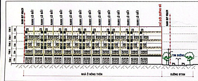
MINH HỌA MẶT ĐŨNG DÂY NHÀ Ở NÔNG THÔN ĐƯỜNG ĐH
