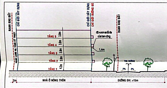
MẶT CẮT QUY ĐỊNH QUẢN LÝ XÂY DỰNG ĐỐI VỚI CÁC DÂY NHÀ MẶT TIỀN ĐƯỜNG ĐH
